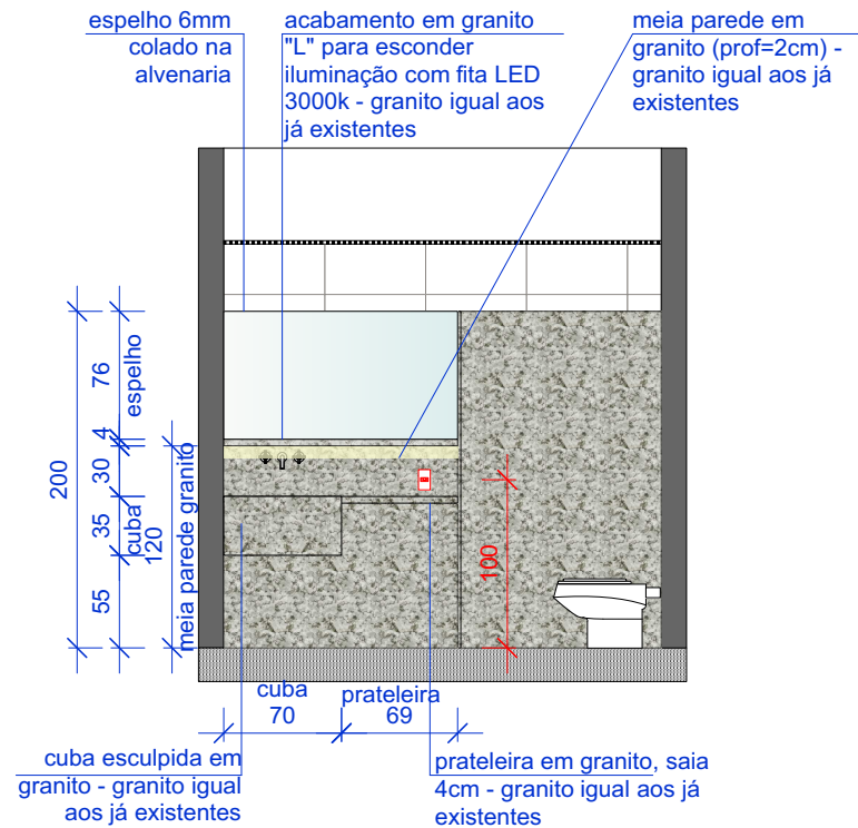
Vista A Escala: 1:50
