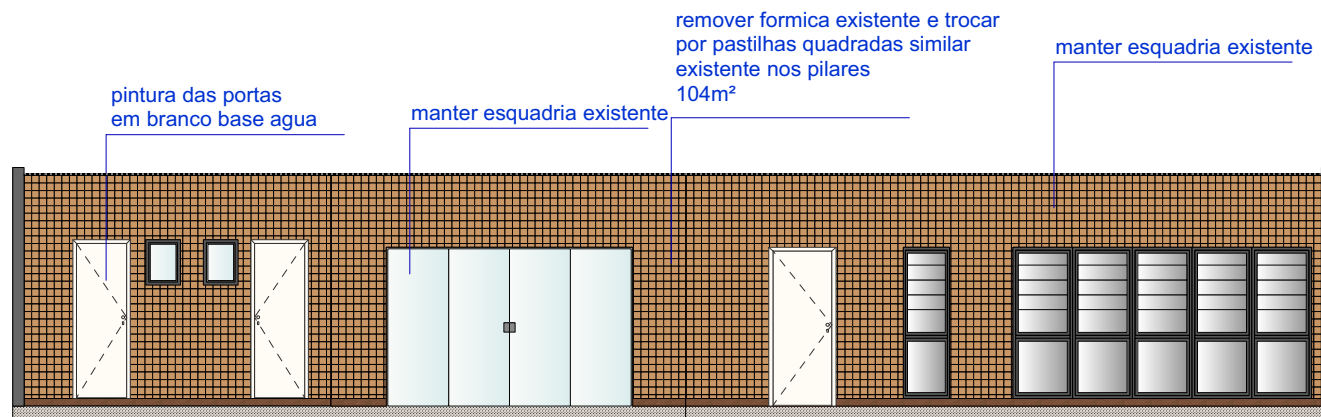
Vista D Escala: 1:100
